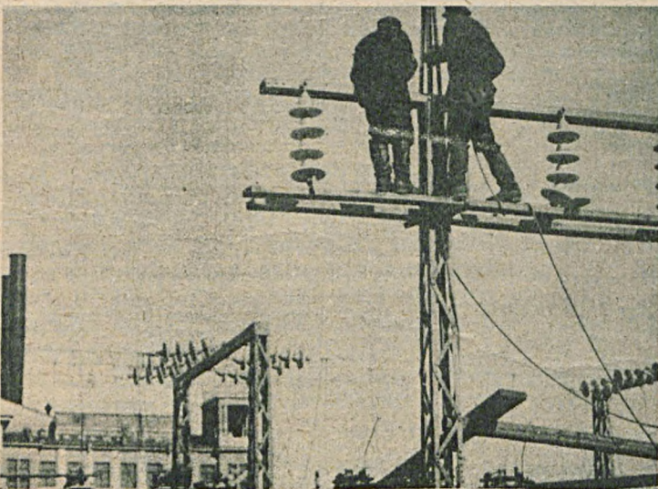
С 1-го мая начала работать Саратовская районная электростанция, с первоначальной мощностью в 11.000 квт. К концу пятилетки общая мощность Саргрэса будет доведена до 40.000 квт. На снимке: последние работы по оборудованию воздушной усилительной подстанции Саргрэса Фот. З. Чеботаева
