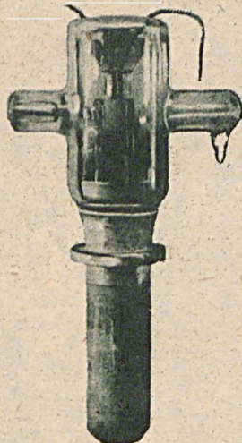
15-киловаттный излучатель ультракоротких волн. С помощью которого проф. Уитней произвел свой знаменитый опыт
