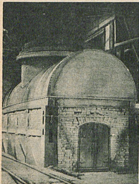
Ватер-жакетная печь для плавки медного колчедана
